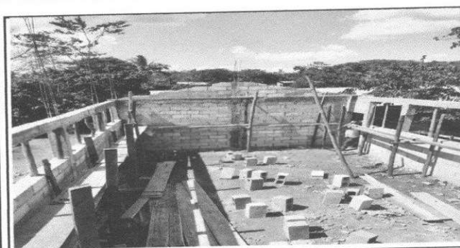
Foto 5: Se observa un 50% del avance del trabajo de la cocina.
